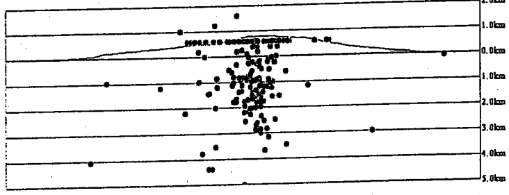
震源分布図 ( 2000年7月4日~7月20日 )
