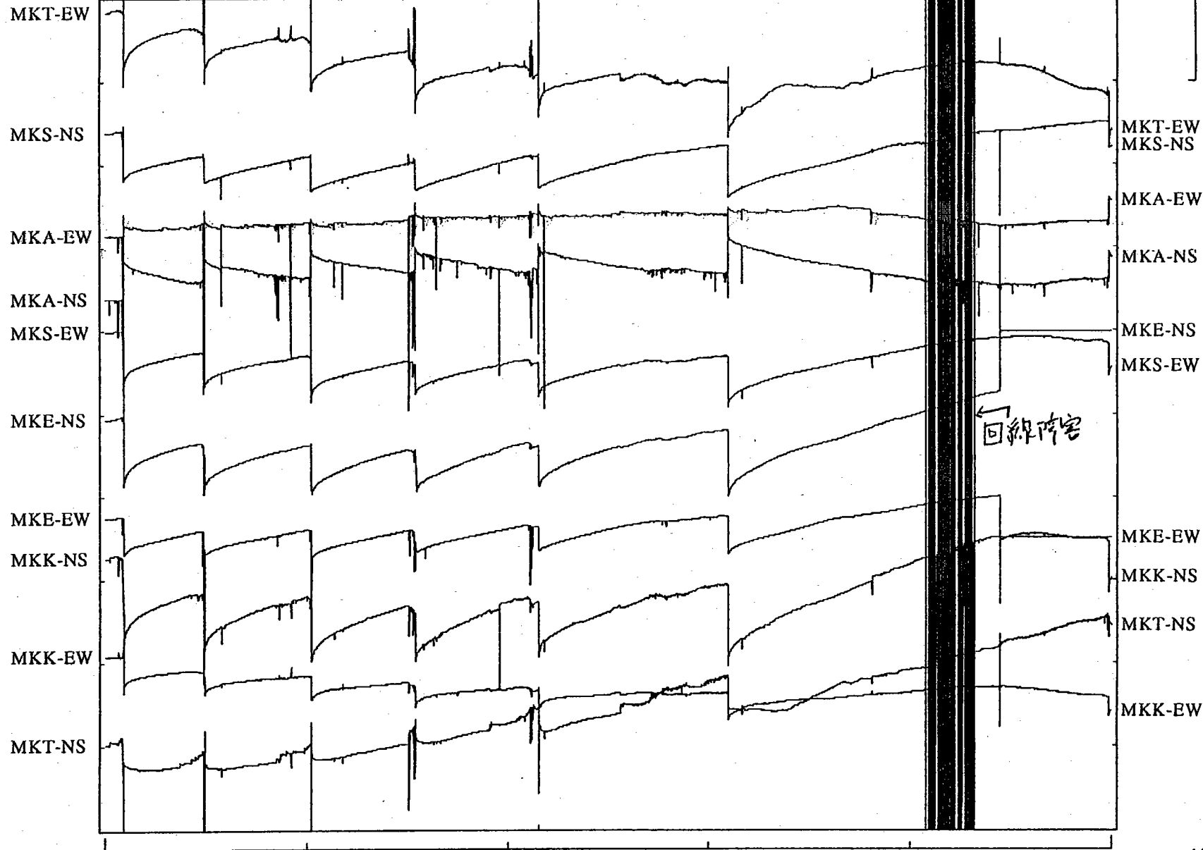
三宅島傾斜変化 (7月11日~7月15日) (資料1「三宅島傾斜変化」の詳細1)
