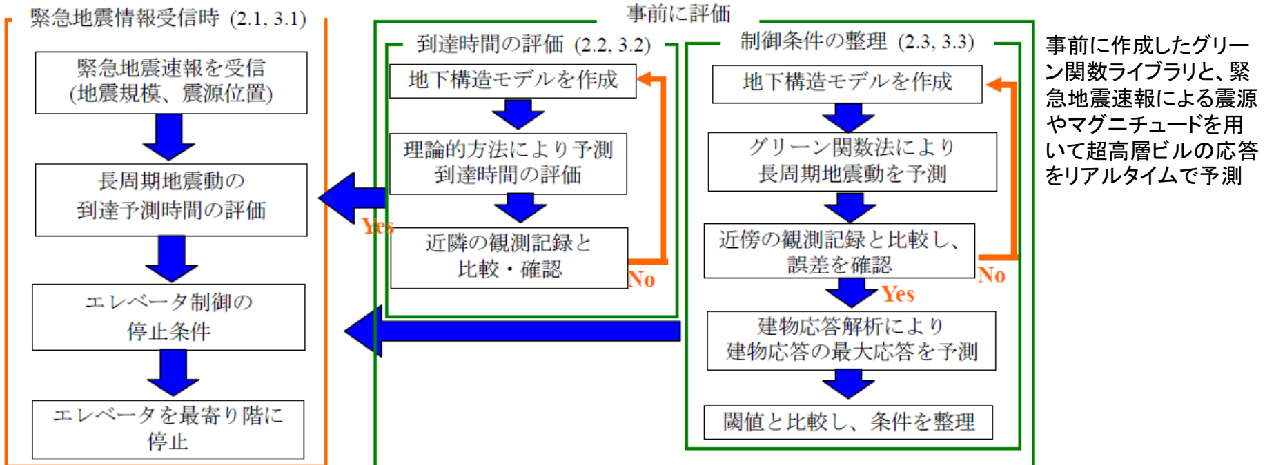
図1：長周期地震動を対象としたエレベータ制御のフロー図
