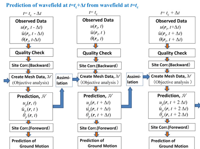
図 1. 実時間地震動予測の処理の流れの概念図.
