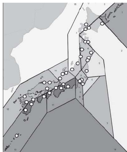
図1 用いた地震地体構造区分 12) と観測点（気象官署）
