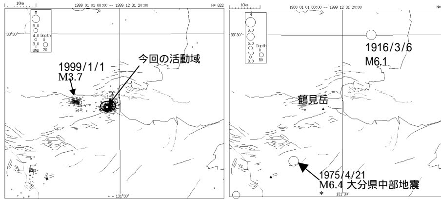
現状 地震活動状況の解説
