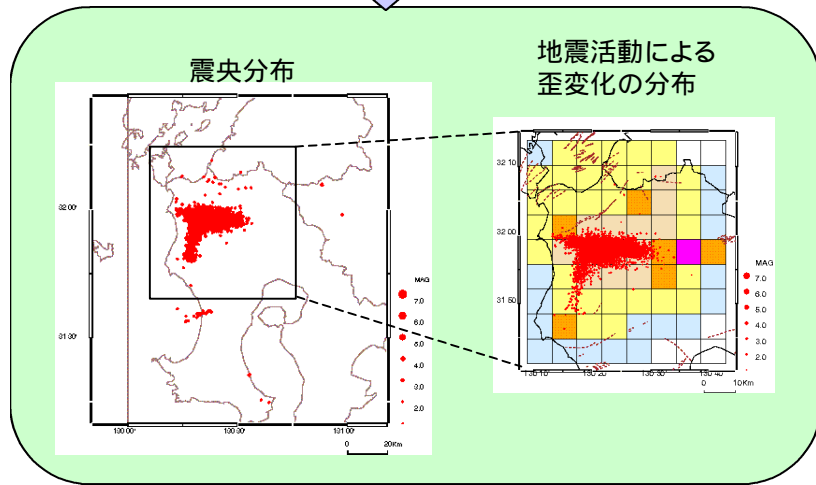
地震活動・地殻の歪等の状態を把握 活動の異常の程度を診断
