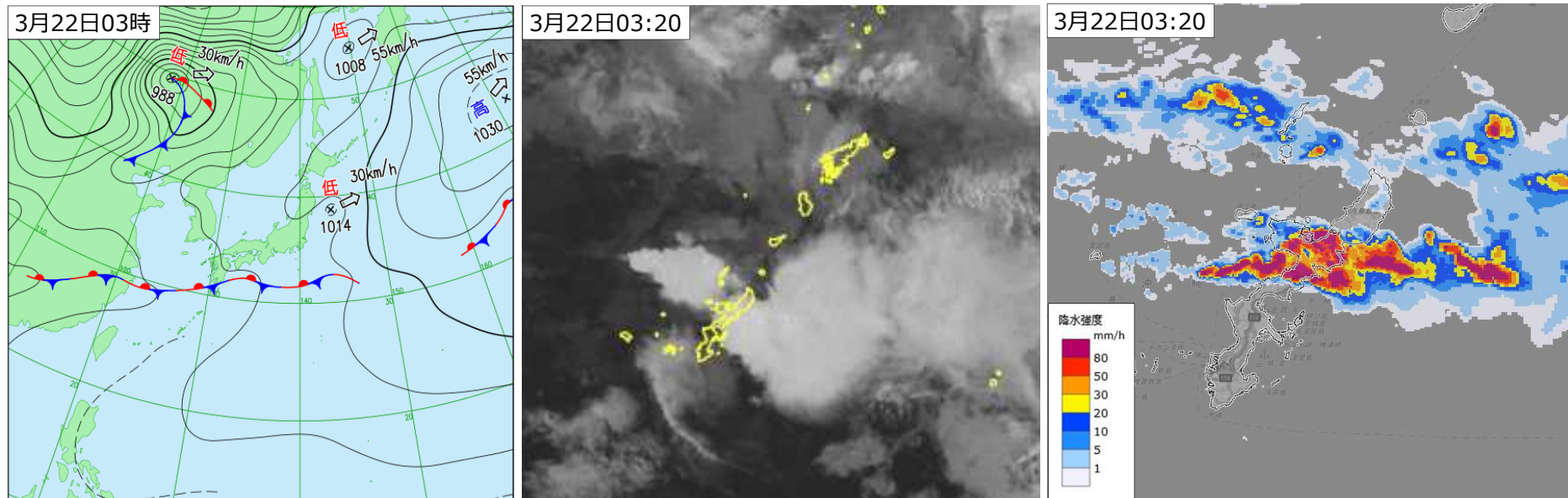
3月22日に沖縄地方で線状降水帯が発生した際の気象状況 左：天気図 中央：気象衛星画像 右：気象レーダー
