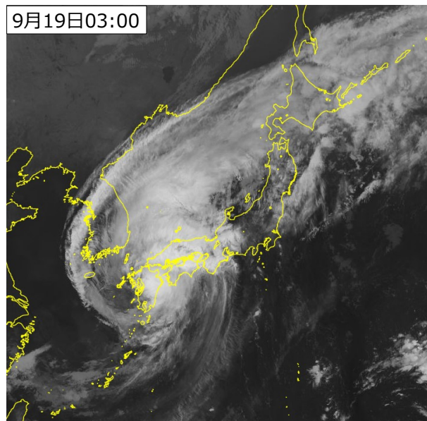
9月19日未明に四国地方で3時間に約150ミリの雨が降った際の気象状況 左:天気図、中央:気象衛星画像、右:気象レーダー
