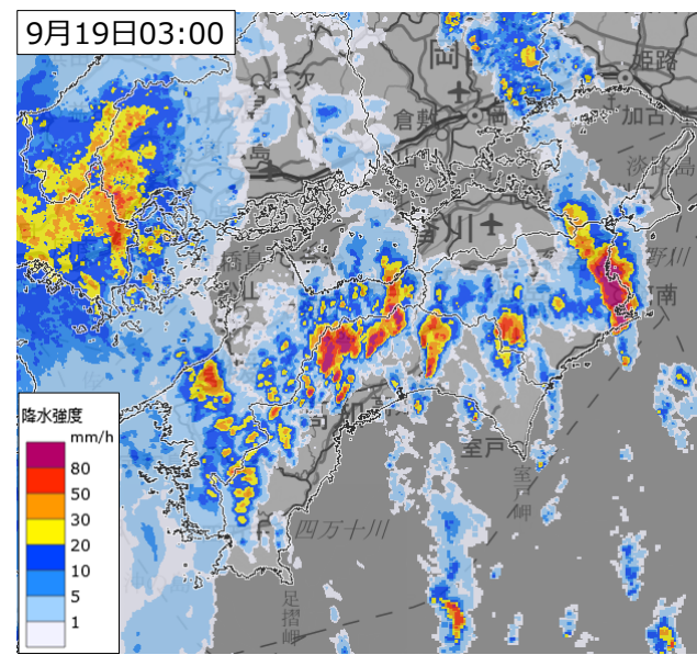
9月19日未明に四国地方で3時間に約150ミリの雨が降った際の気象状況 左:天気図、中央:気象衛星画像、右:気象レーダー
