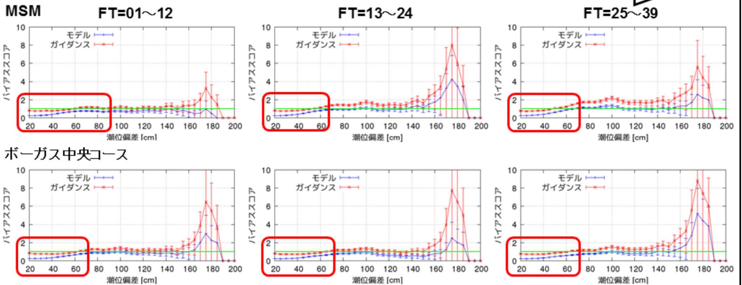
図4.13 高潮予測計算のバイアスコア
