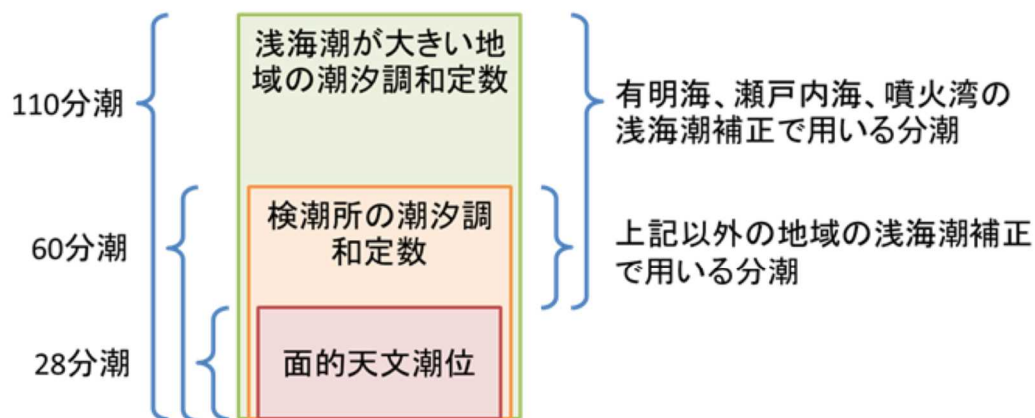
図4.9 浅海潮の補正
