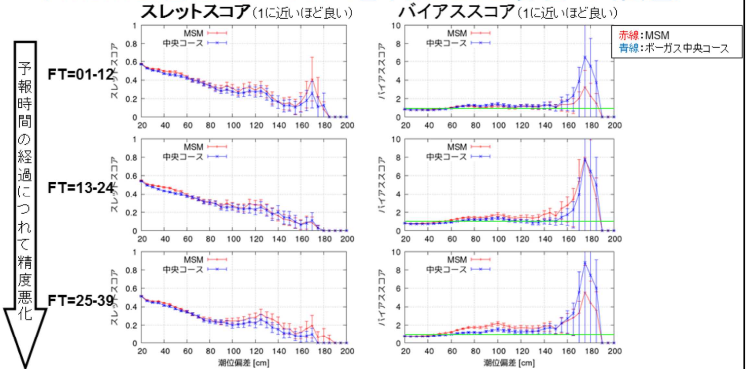
図4.18 高潮ガイダンスによる高潮予測計算の統計スコア(スレットスコア、バイアススコア)
