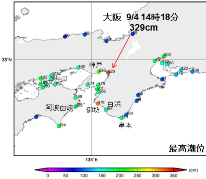
図5.1 台風第21号通過前後で観測された、期間最高潮位(左)と最大潮位偏差(下)
