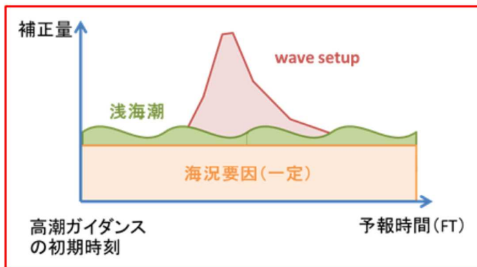
図4.1 高潮モデルの補正のイメージ
