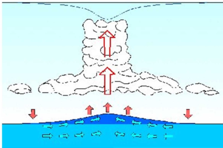
図2.2 吸い上げ効果のイメージ
