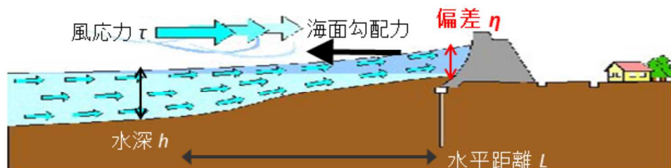
図2.3 吹き寄せ効果のイメージ
