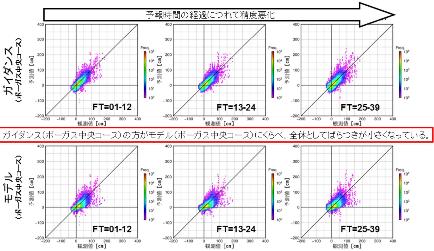
図4.12 潮位偏差観測値(X軸)と予測計算(Y軸)の散布図 統計期間は2019年7月～2021年10月で、台風接近・通過時の事例を抽出した。上段はガイダンス(ボーガス中央コース)、 下段はモデル(ボーガス中央コース)。用いた観測値は図4.11に同じ。
