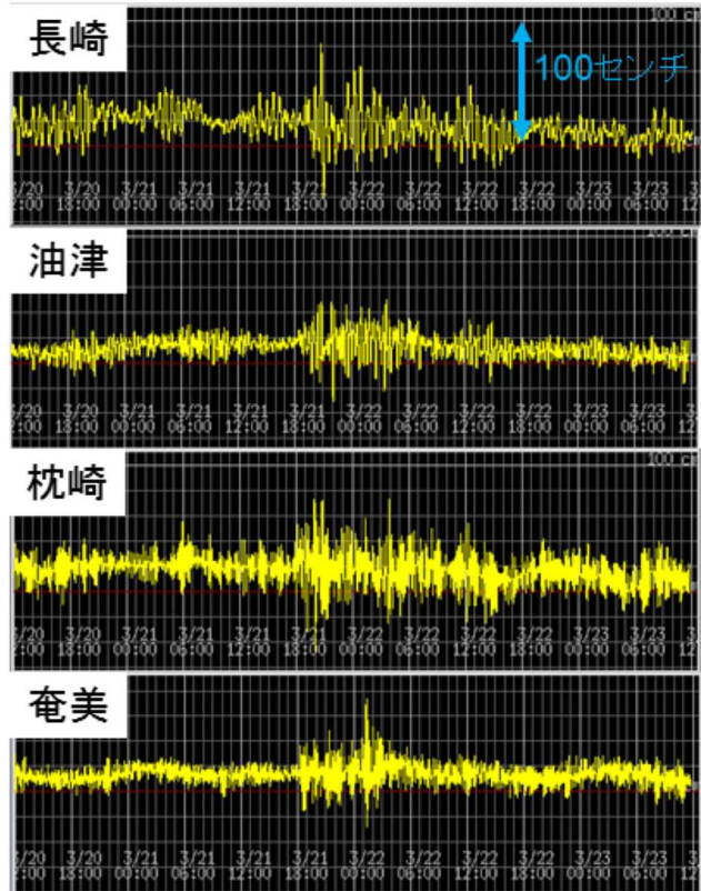
図4.23 2019年3月20～23日に九州、奄美を中心に顕著な副振動が発生した時の潮位偏差
