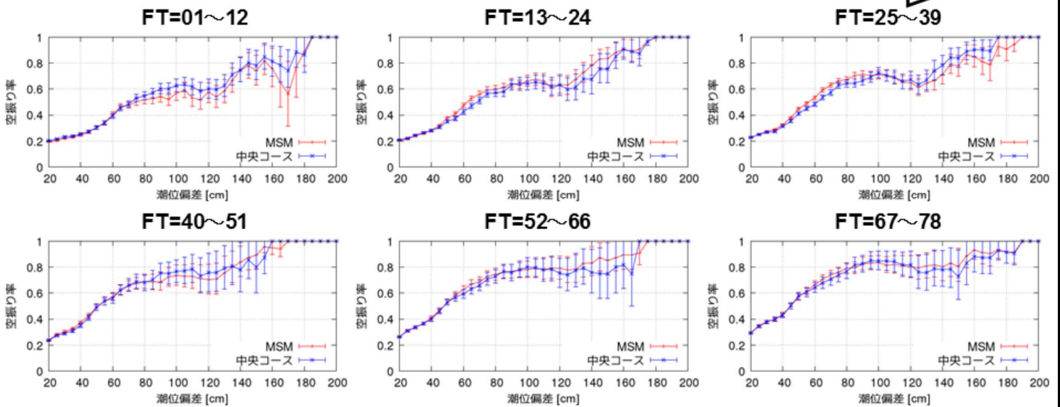
図4.31 高潮ガイダンスによる高潮予測計算の統計スコア(空振り率)
