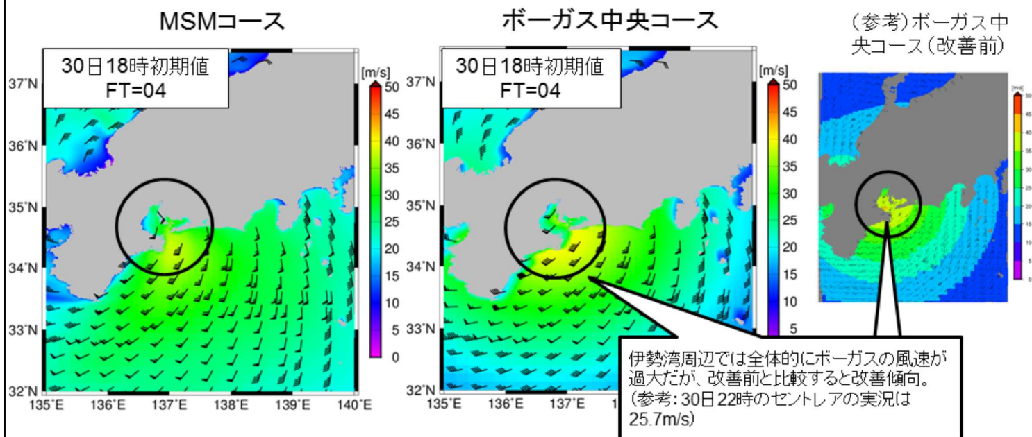
図5.10 30日22時における東海地方周辺の風向風速分布 30日18時(09UTC)初期値のFT=04のプロット。カラーは風速(m/s)、矢羽は風向風速を示す。 左: MSMコース、右: ボーガス中央コース
