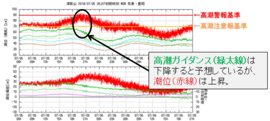
図4.27 2018年7月5日～6日にかけての津居山検潮所の潮位変動(兵庫県による観測)
