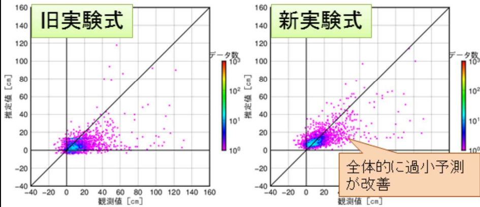
(左) 図4.7 旧実験式(左)及び新実験式(右)を用いた高潮ガイダンス(ハインドキャスト)の散布図。横軸は観測値、縦軸は予測値。検証期間は2019年6月～2021年12月。地点はWave Setup補正量計算地点のみ。3時間最大値で比較。
