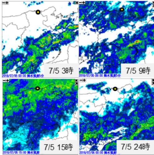
図4.26 2018年7月5日の降雨(黄色丸:津居山検潮所の位置を示す)
