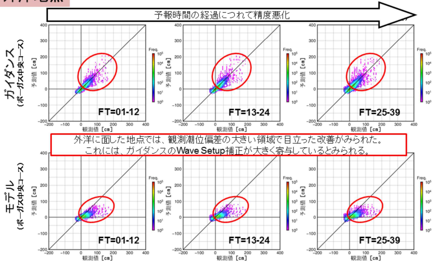
図4.22 外洋地点に対する潮位偏差観測値(X軸)と予測計算(Y軸)の散布図
