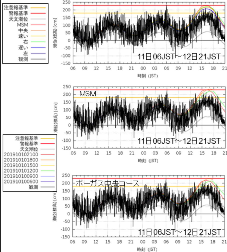
図5.19 三宅島(坪田)の高潮ガイダンス潮位時系列図。上: 11日6時(10日21UTC)初期値における各コースの予測、中: 各初期値のMSMコース、下: 各初期値のボーガス中央コース
