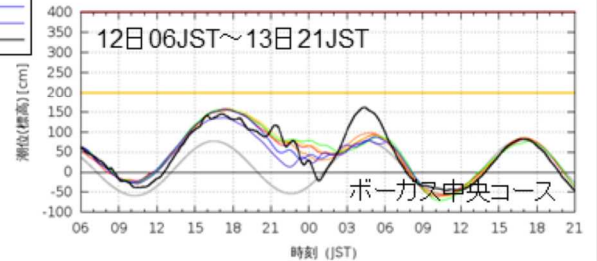
図5.18 東京の高潮ガイダンス潮位時系列図。上: 12日6時(11日21UTC)初期値における各コースの予測、中: 各初期値のMSMコース、下: 各初期値のボーガス中央コース
