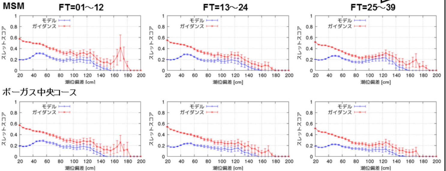
図4.16 高潮予測計算のスレットスコア
