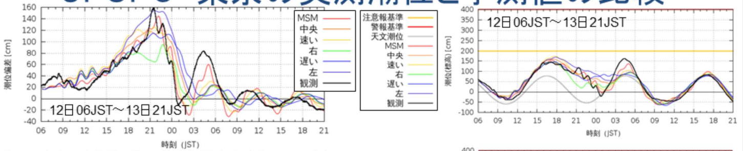
図5.17 東京の高潮ガイダンス潮位偏差時系列図。12日6時(11日21UTC)初期値における各コースの予測
