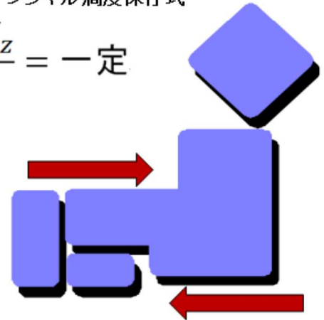
図4.24 陸棚波の伝播イメージ
