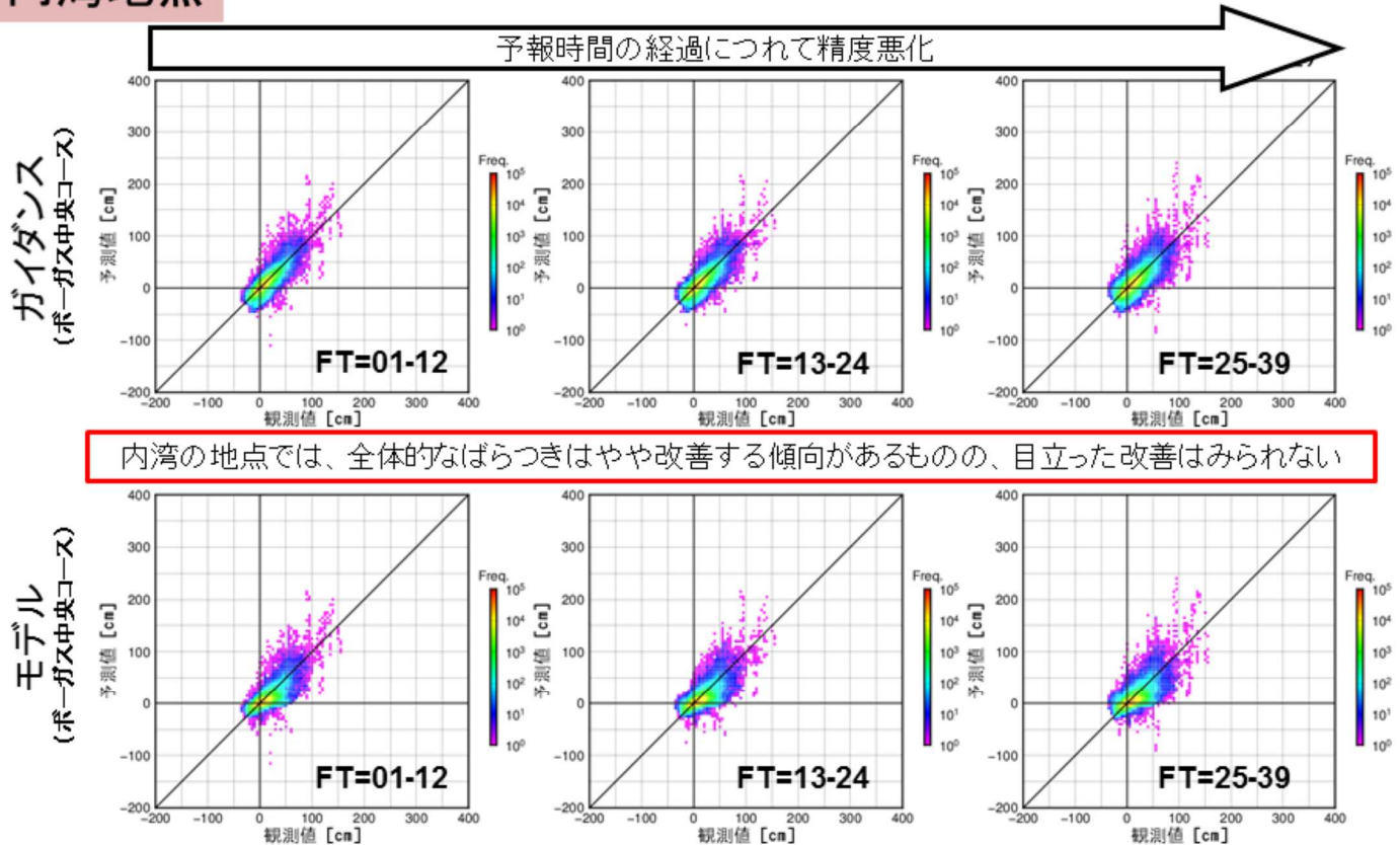
図4.20 内湾地点に対する潮位偏差観測値(X軸)と予測計算(Y軸)の散布図
