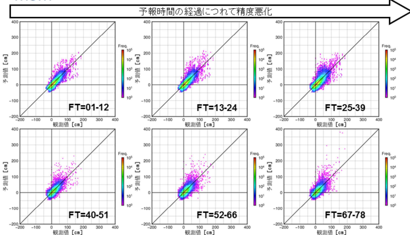
図4.28 高潮ガイダンスによる潮位偏差観測値(X軸)と予測計算(Y軸)の散布図(MSM) 統計期間は2019年7月～2021年10月の台風接近・通過時。用いた観測値は図4.11と同じ。
