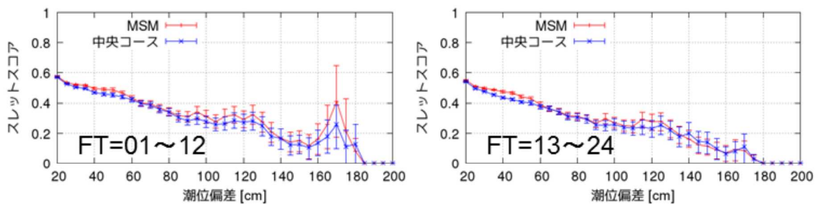
図6.1 高潮ガイダンスによる高潮予測の捕捉率(赤線:MSM、青線:ボーガス中央コース、エラーバーは95%の信頼区間を示す。)図4.18と同じ。
