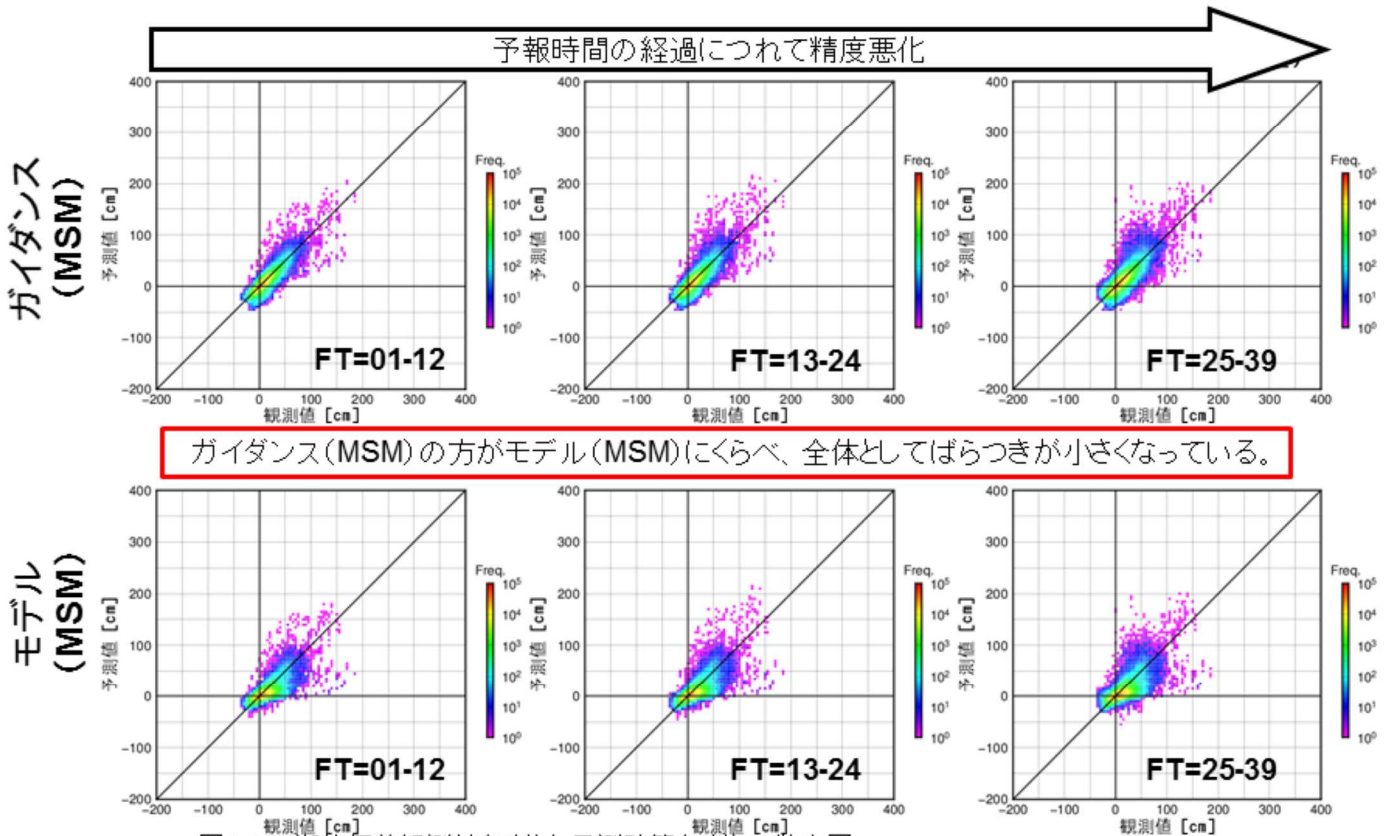
図4.11 潮位偏差観測値(X軸)と予測計算(Y軸)の散布図 統計期間は2019年7月～2021年10月で、台風接近・通過時の事例を抽出(全885初期値)。上段はガイダンス(MSM)、下段はモデル(MSM)を示す。国内約200地点の潮位観測点(気象庁ほか、港湾局や海上保安庁、国土地理院が運用)の観測値を使用し、3時間ごとの最大値で比較。
