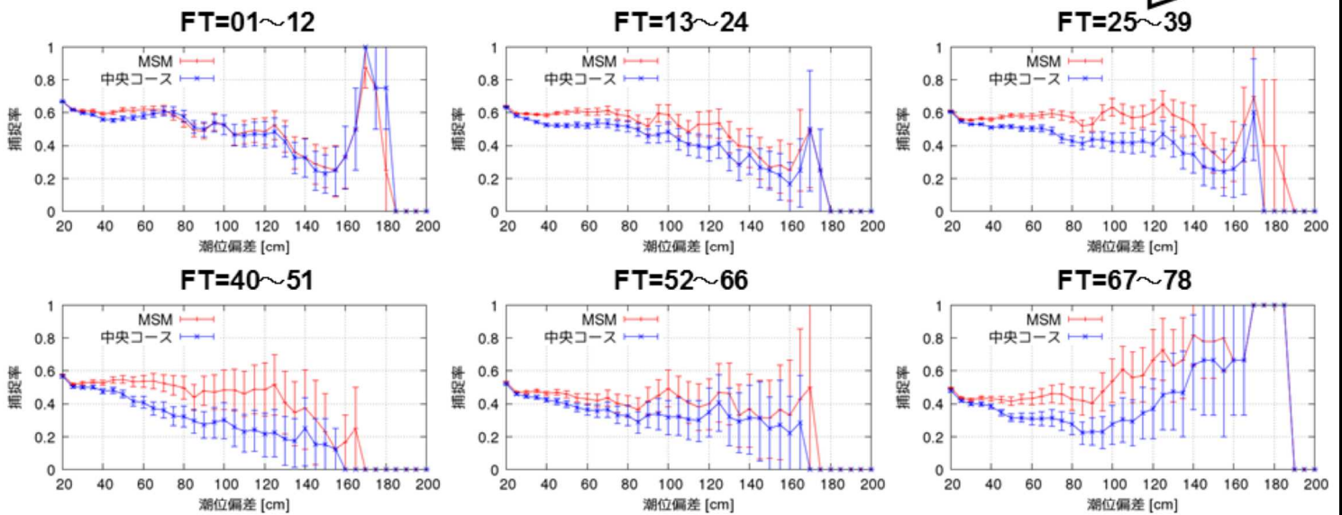
図4.32 高潮ガイダンスによる高潮予測計算の統計スコア(捕捉率)
