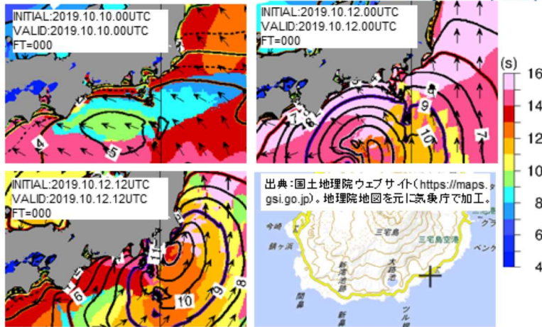
図5.24 沿岸波浪モデルによる10月10日、12日の有義波高(等高線)・波向(矢印)・波の周期(色)と三宅島(坪田)の検潮所位置(図中にて+で表示)
