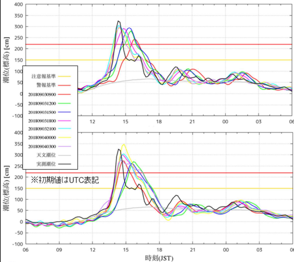
図5.7 大阪での高潮ガイダンスによる各初期値の潮位予想 (上:MSMコース、下:ボーガス中央)
