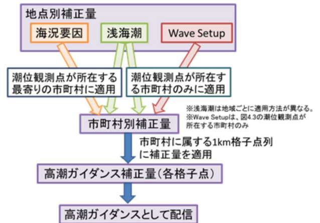
図4.2 高潮モデル補正の流れ
