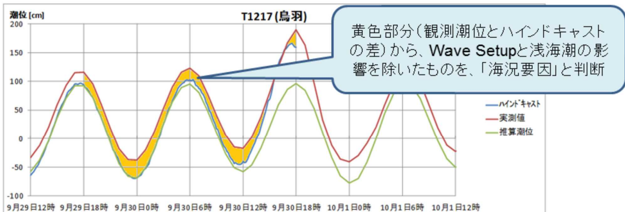
図4.10 海況要因の補正
