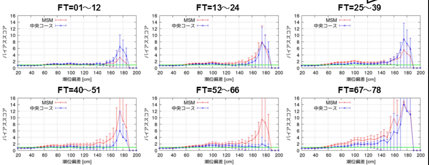
図4.30 高潮ガイダンスによる高潮予測計算の統計スコア(バイアスコア)
