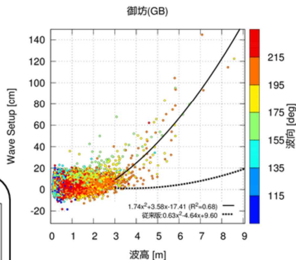
図4.4 御坊における波浪モデルの波高とWave Setup観測値の分布 実線は2023年に導入した実験式で、点線は旧実験式
