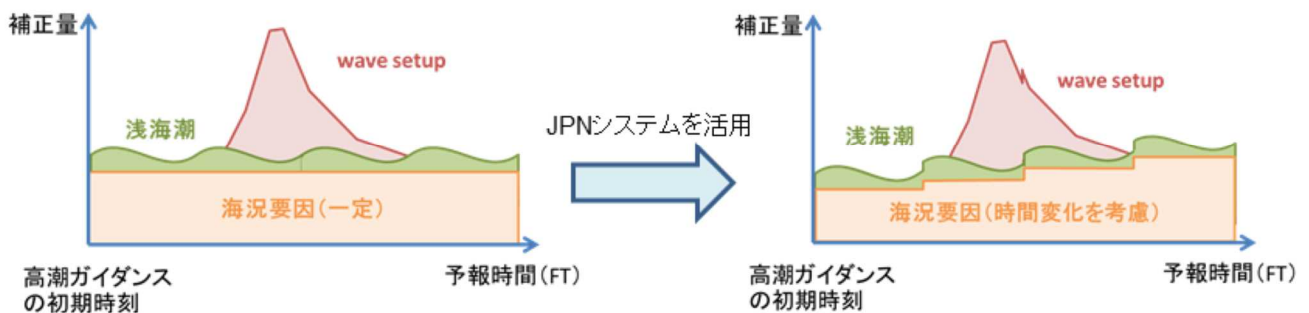
図7.4 補正量算出方法の改善のイメージ(左:現在 右:改善後)
