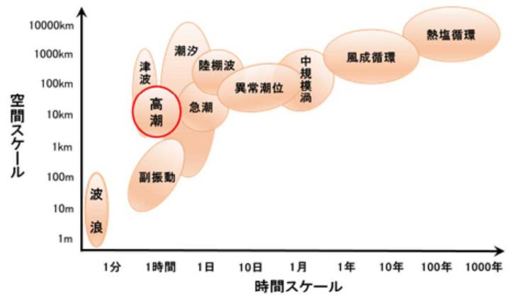
図2.5 海洋現象の時空間スケール
