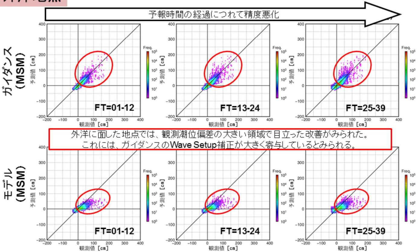
図4.21 外洋地点に対する潮位偏差観測値(X軸)と予測計算(Y軸)の散布図
