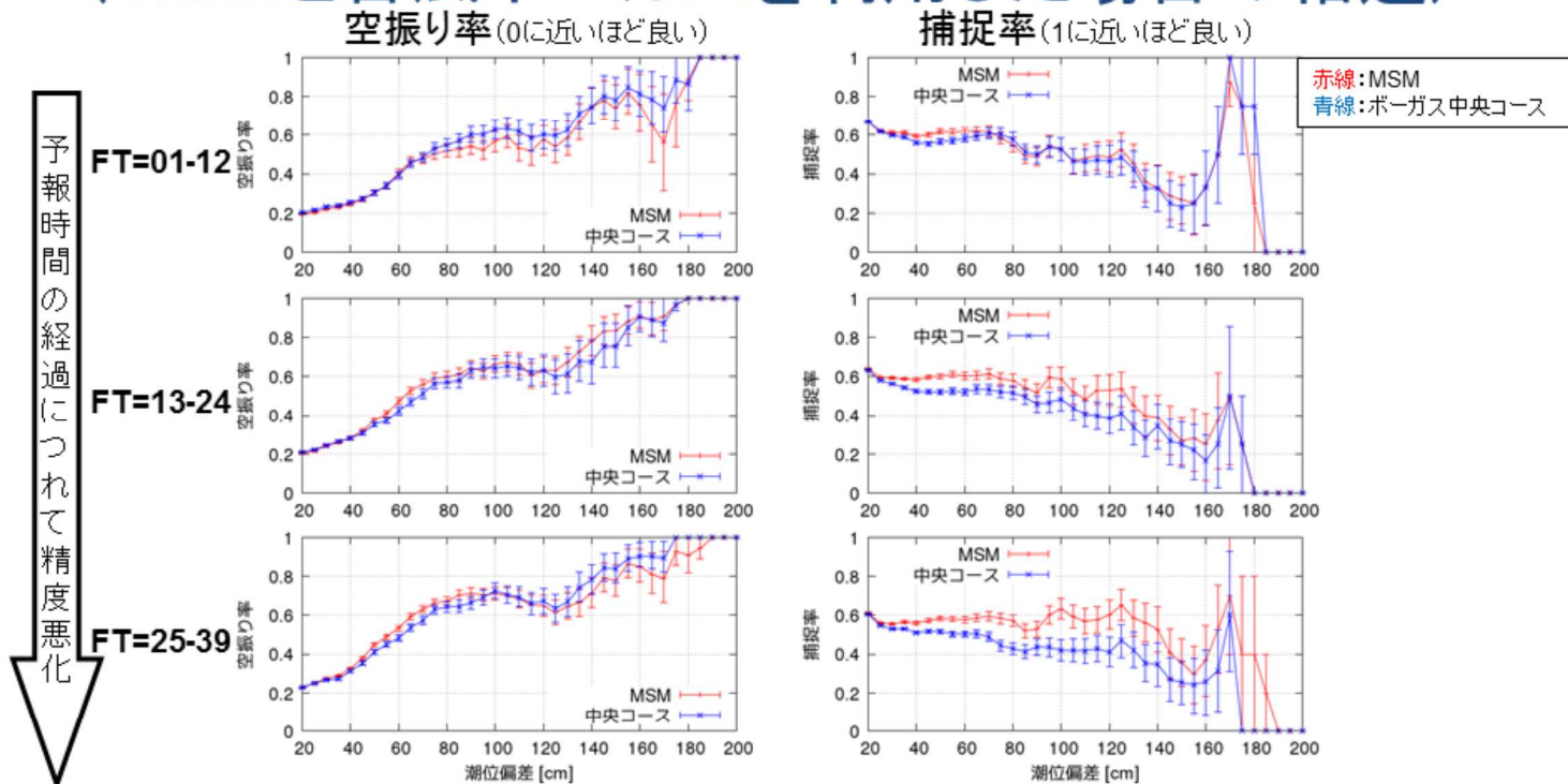
図4.17 高潮ガイダンスによる高潮予測計算の統計スコア(空振り率、捕捉率)
