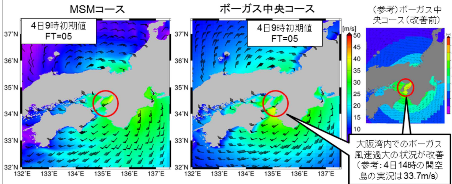
図5.4 4日14時における近畿地方周辺の風向風速分布 4日9時(00UTC)初期値のFT=05のプロット。カラーは風速(m/s)、矢羽は風向風速を示す。 左: MSMコース、中央: ボーガス中央コース(改善後)、右: ボーガス中央コース(改善前)
