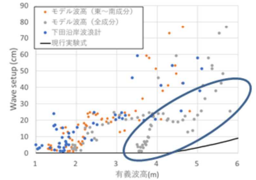
図7.3 令和元年台風第15号で観測された下田沿岸波浪計の波高(青色)、沿岸波浪モデル有義波高(灰色)、東～南成分の有義波高(橙色)に対する石廊崎のWave Setup解析値の散布図
