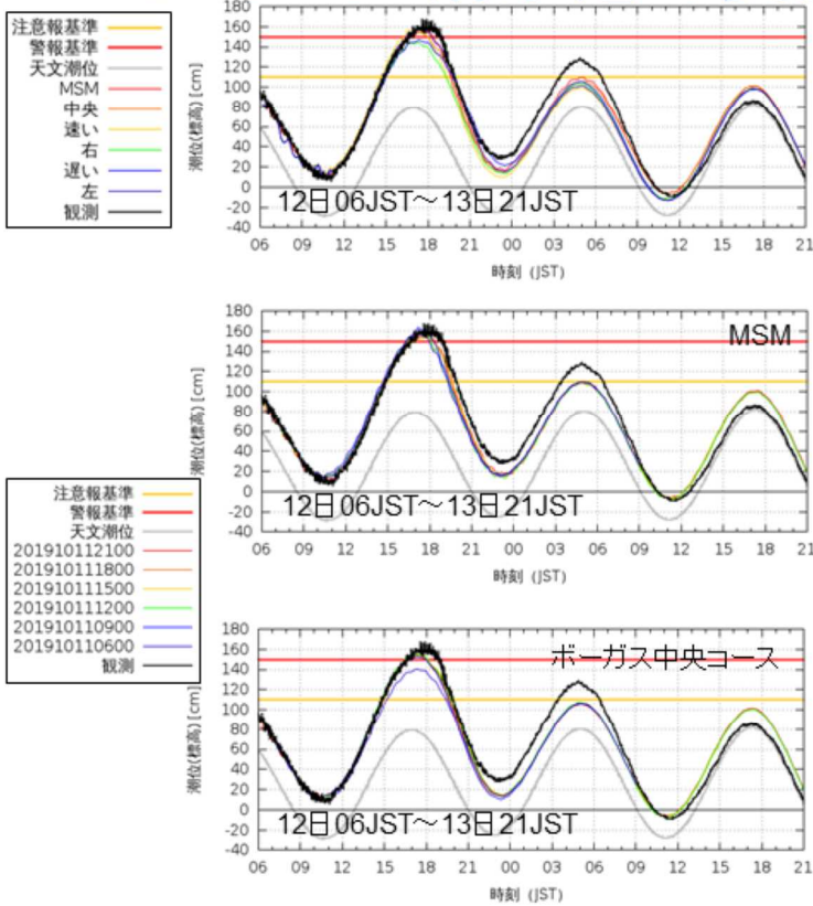
図5.21 清水港の高潮ガイダンス潮位時系列図。上：12日6時(11日21UTC)初期値における各コースの予測、中：各初期値のMSMコース、下：各初期値のボーガス中央コース
