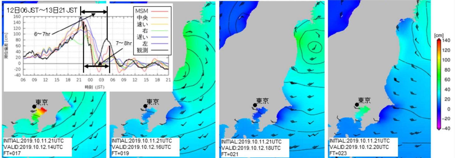
図5.23 MSMコースにおける12日6時(11日21UTC)初期値の潮位偏差予想(FT=17, 19, 21, 23)と東京の高潮ガイダンス潮位偏差時系列図。時系列図中の各コースの予測は12日6時(11日21UTC)初期値によるもの
