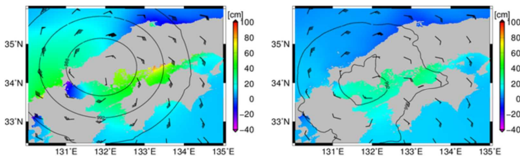
図6.2 ポーガス中央コース(左)とMSM(右)それぞれでの風・気圧・潮位偏差の分布図(カールスケールは潮位偏差のもの)。20180728 18UTC初期値 (FT=12)の結果
