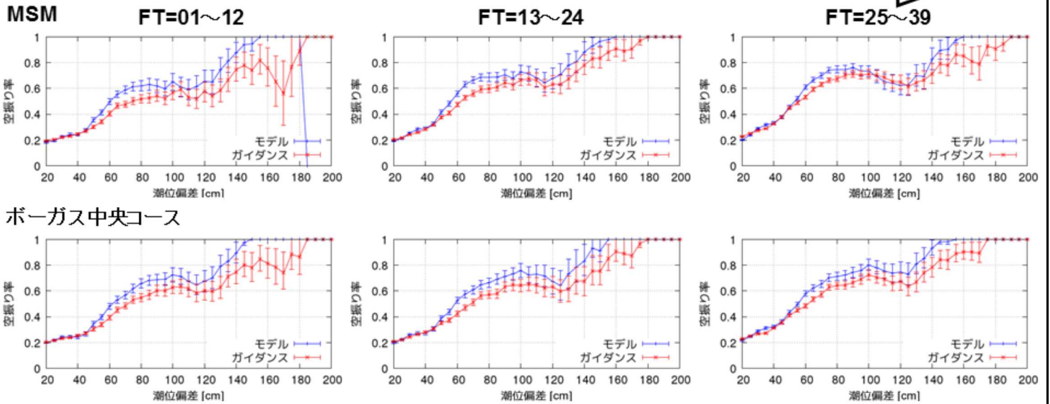
図4.14 高潮予測計算の空振り率
