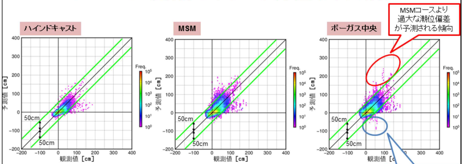
図3.3 日本域高潮モデルのハインドキャスト(左)、MSMコース(中)、及びボーガス中央コース(右)における潮位偏差観測値(X軸)とモデル計算(Y軸)の散布図。検証期間、観測値、中図と右図の予報時間は図3.1と同じ。
