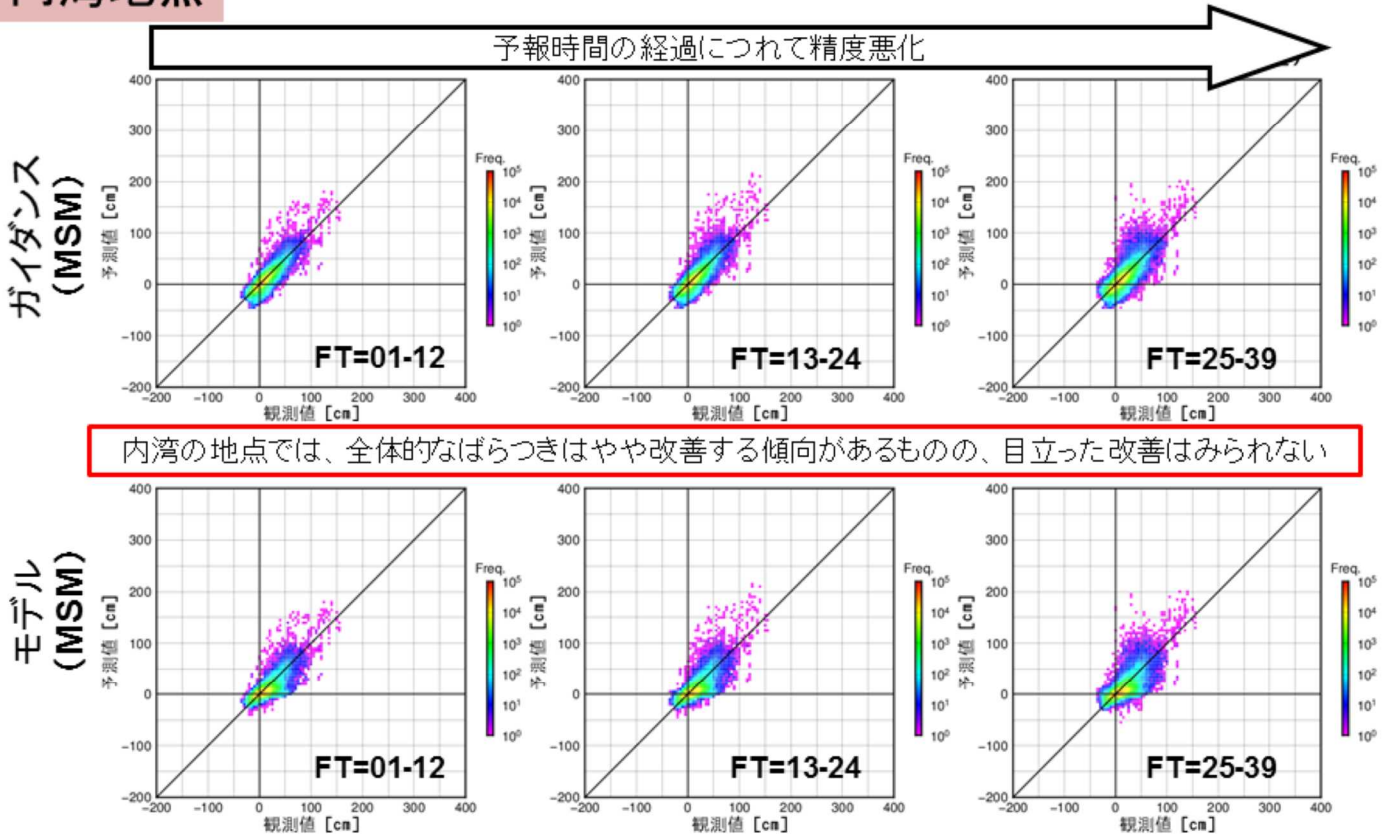
図4.19 内湾地点に対する潮位偏差観測値(X軸)と予測計算(Y軸)の散布図
