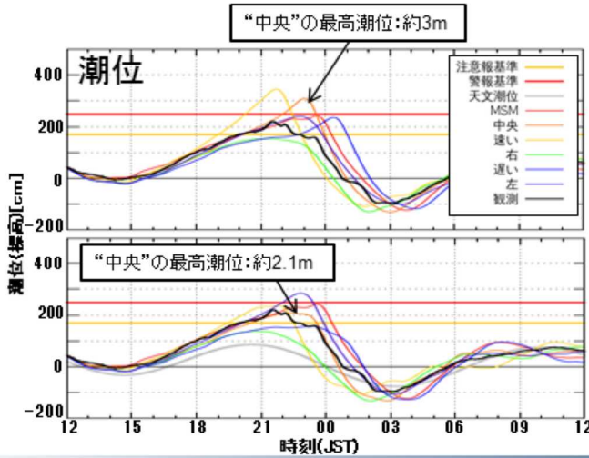
図5.13 30日3時 初期時刻 予想
