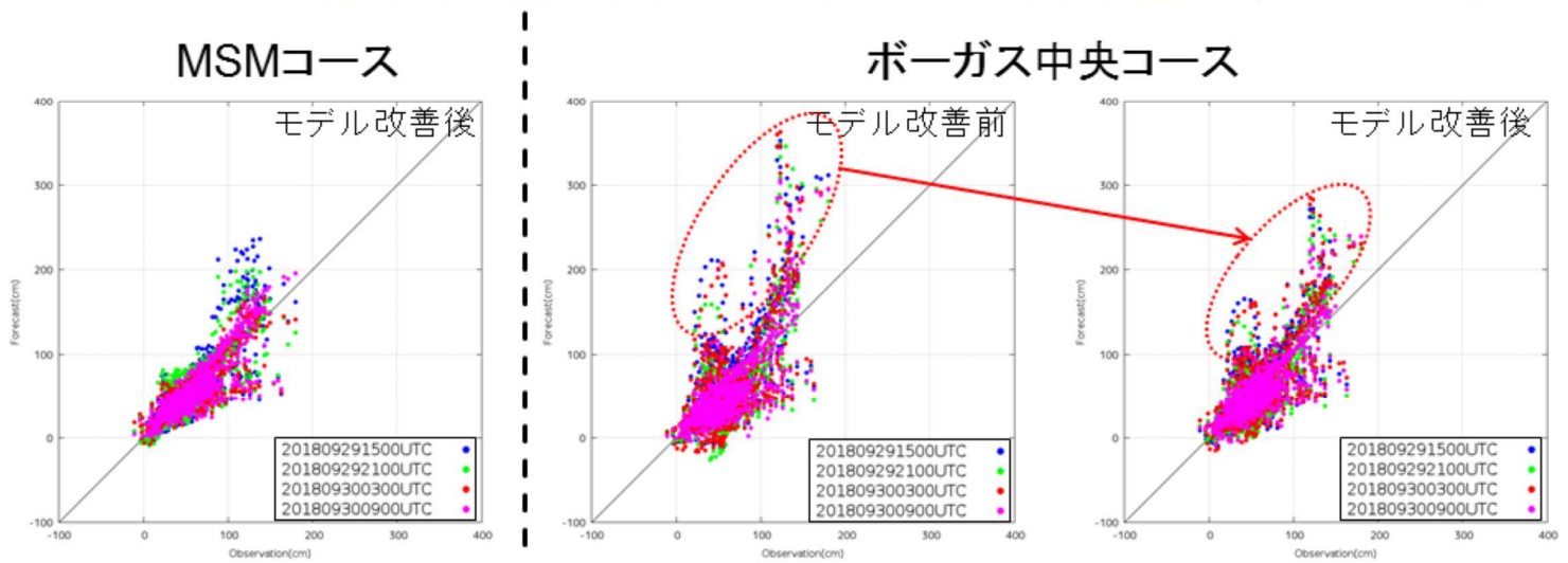
図5.9 高潮ガイダンスについて、近畿～東海地方周辺の30日0時(29日15UTC)～30日18時(09UTC)まで6時間ごとの初期値のプロット。大きめの潮位偏差が観測された30日17時(08UTC)～10月1日00時(9月30日15UTC)までの時間帯に絞っている。
