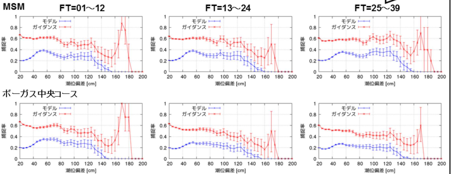
図4.15 高潮予測計算の捕捉率
