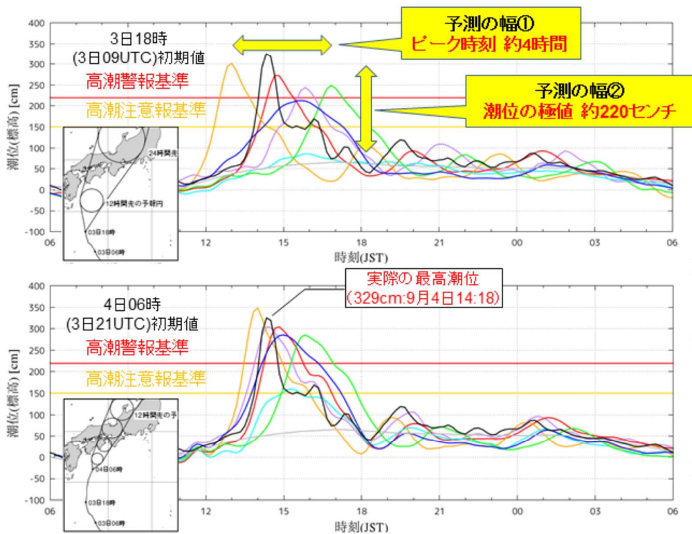
図5.5 大阪での潮位 6コース 高潮ガイダンス潮位データ 上図は3日18時(3日09UTC)、下図は4日06時(3日21UTC)初期値
