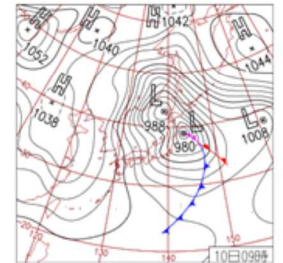
図4.5 2015年3月10日09時の地上天気図
