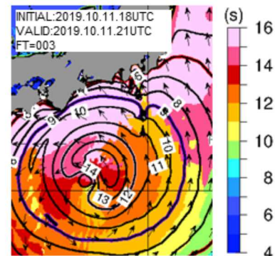
図5.20 沿岸波浪モデルによる12日6時(11日21UTC)における有義波高(等高線)・波向(矢印)・波の周期(色)
