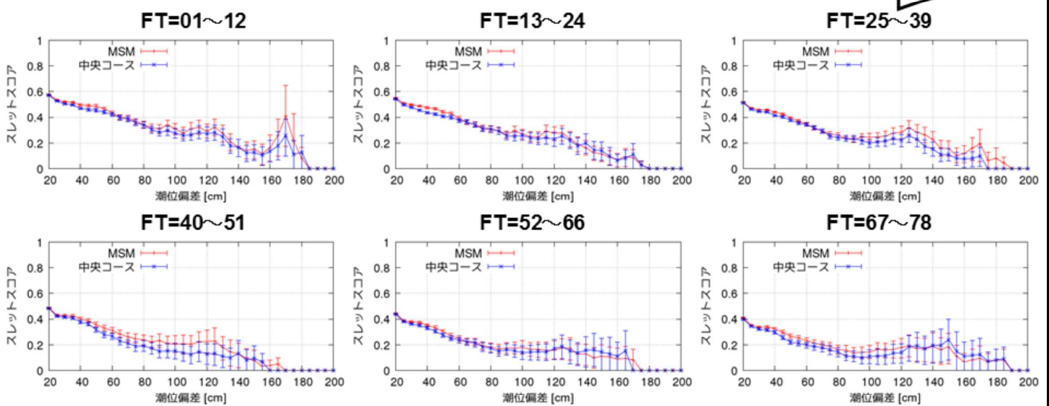
図4.33 高潮ガイダンスによる高潮予測計算の統計スコア(スレットスコア)
