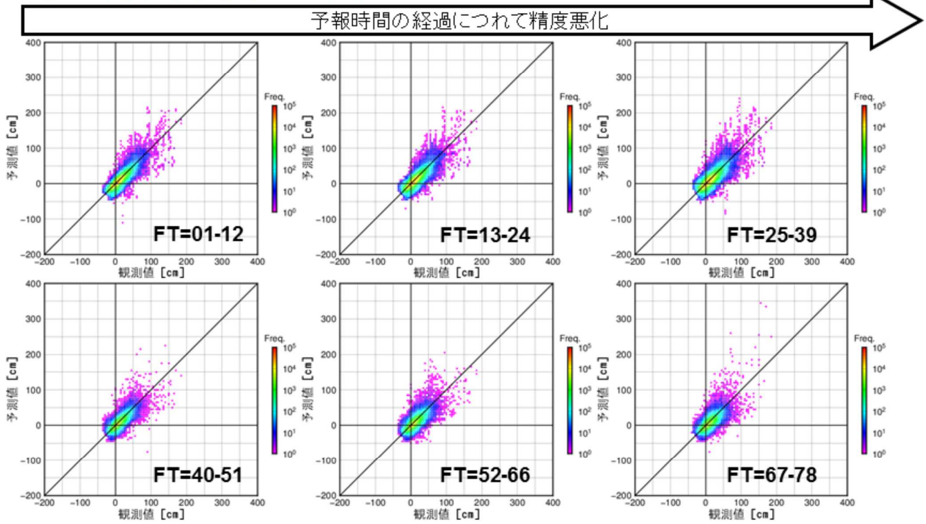
図4.29 高潮ガイダンスによる潮位偏差観測値(X軸)と予測計算(Y軸)の散布図(ボーガス中央コース) 統計期間は2019年7月～2021年10月の台風接近・通過時。用いた観測値は図4.11と同じ。
