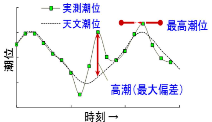
図2.1 潮位、高潮のイメージ
