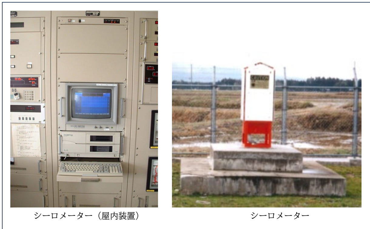
図 3-2-2 空港気象常時監視通報装置、空港気象常時監視装置（3/3）
