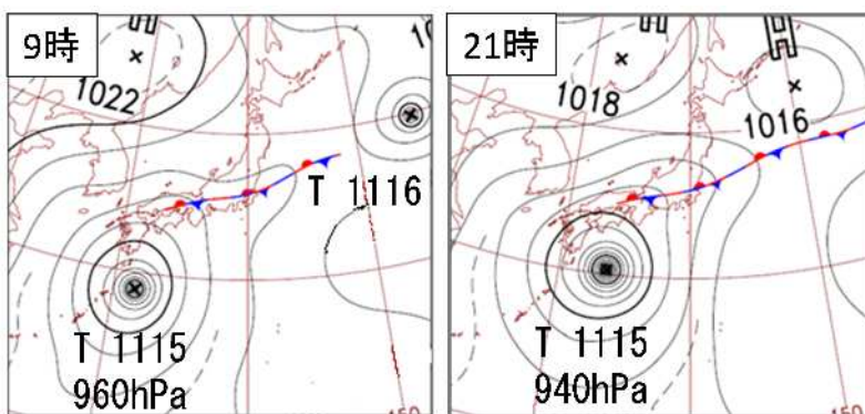
第 1.2.1.1 図 9 月 20 日の地上天気図
