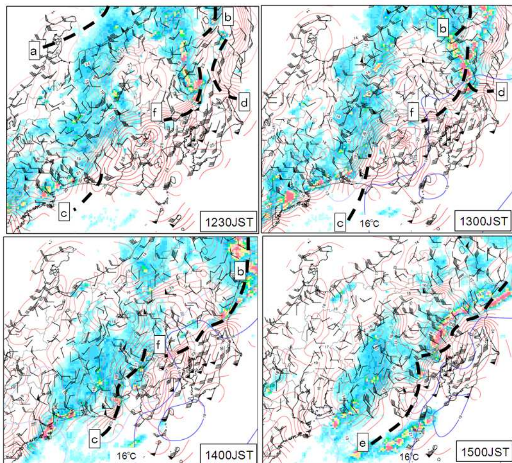
1.3.1.17 図 局地解析図（6日 1230JST～1500JST）
