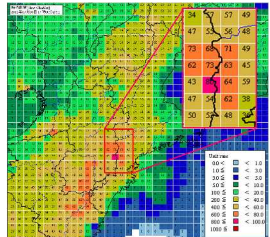
第 1.2.2.12 図 最大 1 時間解析雨量 (2012 年 9 月 30 日 15 時)
