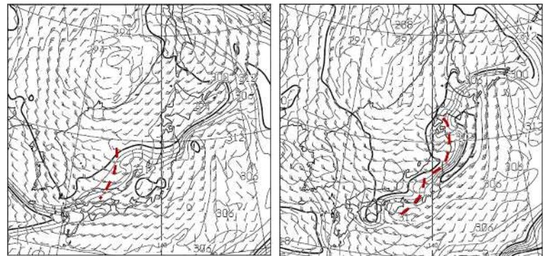
第 1.3.1.7 図 GSM850hPa 風・相当温位予想図 （5 日 12UTC 初期値、左図：6 日 09JST 予想、右図：21JST 予想） 短矢羽根：5kt、長矢羽根：10kt、ペナント：50kt、茶破線：シアー
