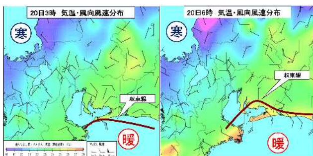
第1.2.1.20図 20日3時と6時の地上分布図
