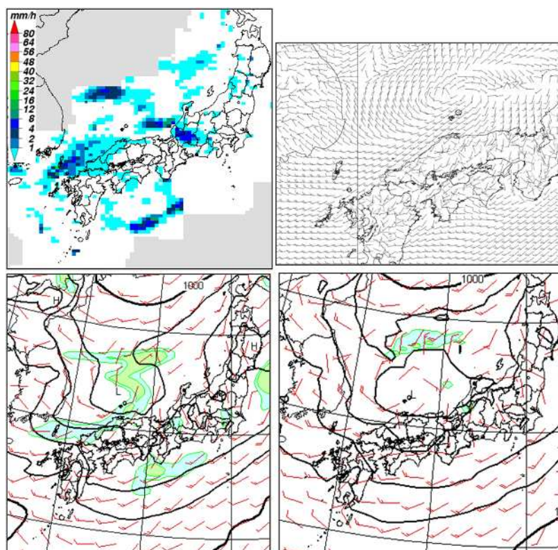
第 1.3.1.14 図 実況とモデルの比較（6日 03JST）
