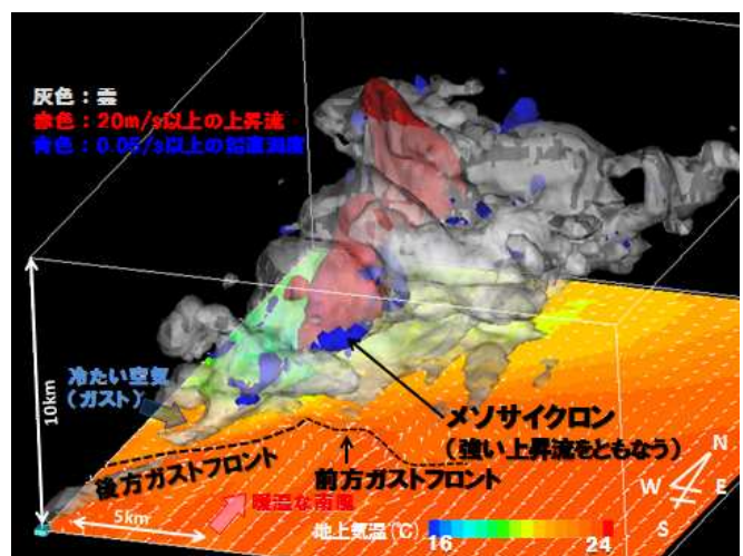
第 1.3.3.7 図 水平解像度 250m の数値シミュレーションで再現されたつくば竜巻をもたらしたスーパーセル 灰色は雲、赤色は強い上昇流、青色は強い鉛直渦度の領域を示す。
