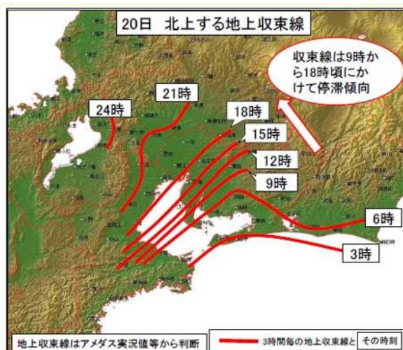
第 1.2.1.14 図 20 日の北上する地上収束線
