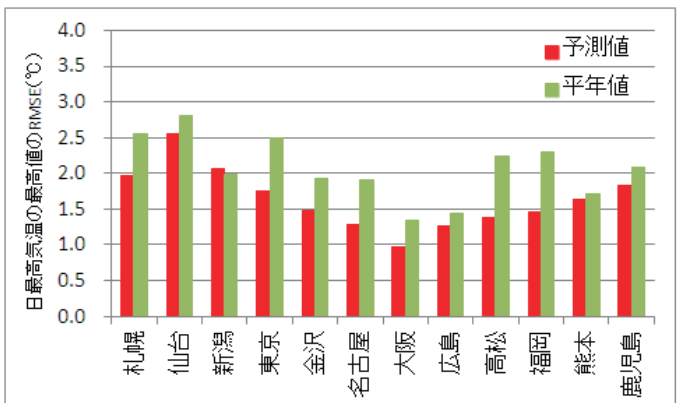
第 2.3.3.5 図 2 週目の日最高気温の RMSE(単位℃)
