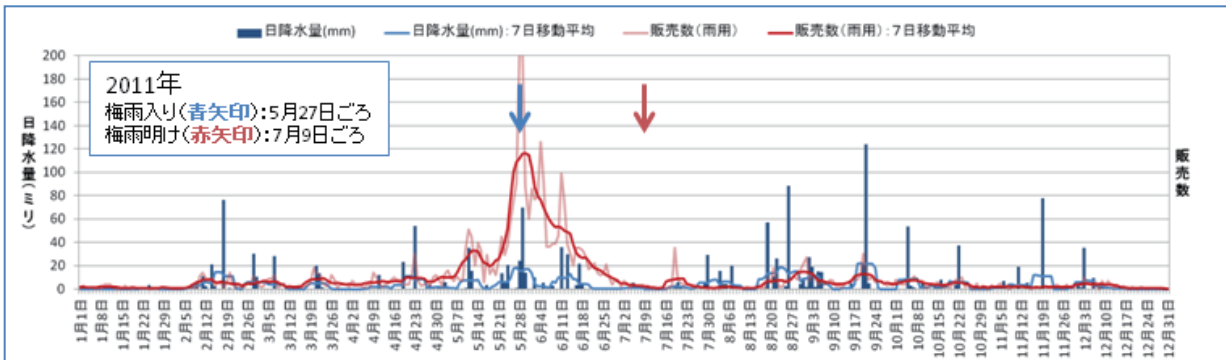
第 2.3.4.6 図 雨用靴の販売数と降水量との関係 アパレル・ファッション産業分野における気候リスク評価調査報告書より抜粋
