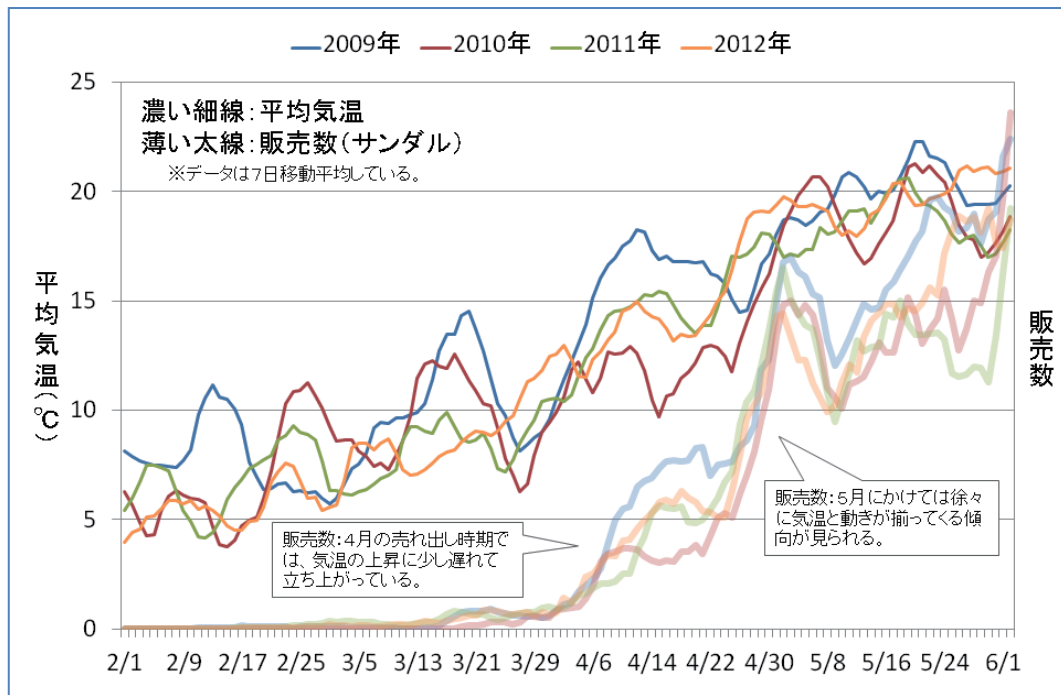
第 2.3.1.15 図 サンダルの販売数と気温の時系列グラフ
