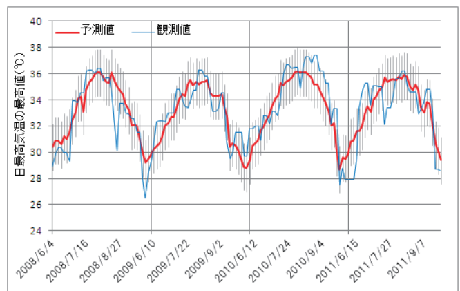
第2.3.3.3図 日最高気温の最高値の予測(大阪) 横軸：予測期間の初日の日付 縦軸：日最高気温の最高値(°C) 赤実線は予測値、青実線は観測値を表す。 灰色の縦線は予測の80%信頼幅を表す。
