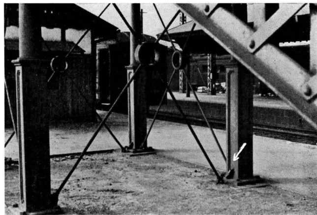
(10) 關西線王寺驛陸橋下筋違ひ(北側)鐵棒の切斷
