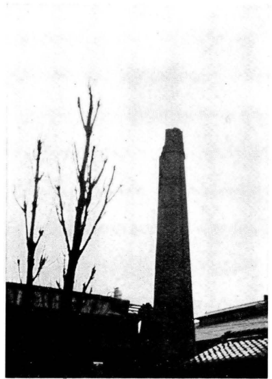
(4) 奈良縣磯城郡川西村梅戸の膠工場の 煙突 (基部の徑2.4 米, 高さ 約21 米) 上部の破損
