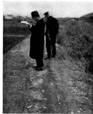
(15) 王寺驛南方500m 葛下川 北側堤防上の龜裂(幅 2cm, 長さ15m)。
