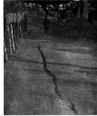
(3) 高田公園池畔道路の龜裂 (方向は南北で幅3cm, 長さ6m)。
