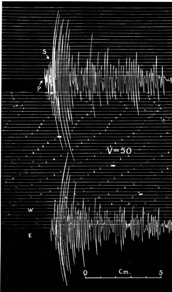
河内大和強震地震計記象 (其の1) 洲本 水平動 (簡單微動計) 上下動 (ウキーヘルト式)
