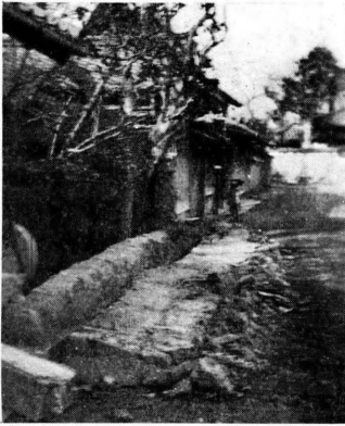
(7) 瀬南村南郷の土塀(幅 30 cm, 高さ 1.3m, 長さ 7m) 北側へ倒壊す。
