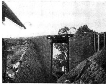
(1) 大鐵柏原南口驛北東陸橋石臺の崩れ。東側より見る。(左圖参照)
