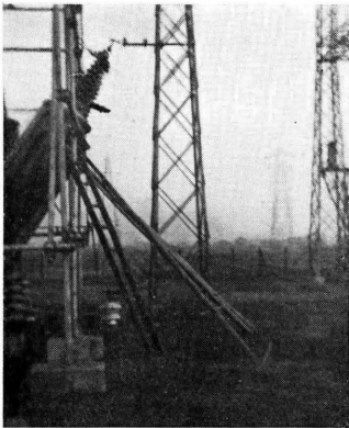
(4) 高田變電所「アルミニュー ム, アレスター」徑70cm, 長さ3mのもの東側へ傾斜。
