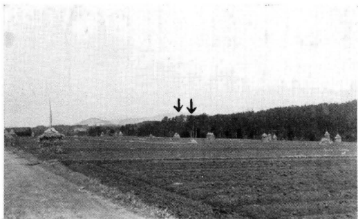
(6) 發光現象を見たと言はれる山を現場より撮す。
