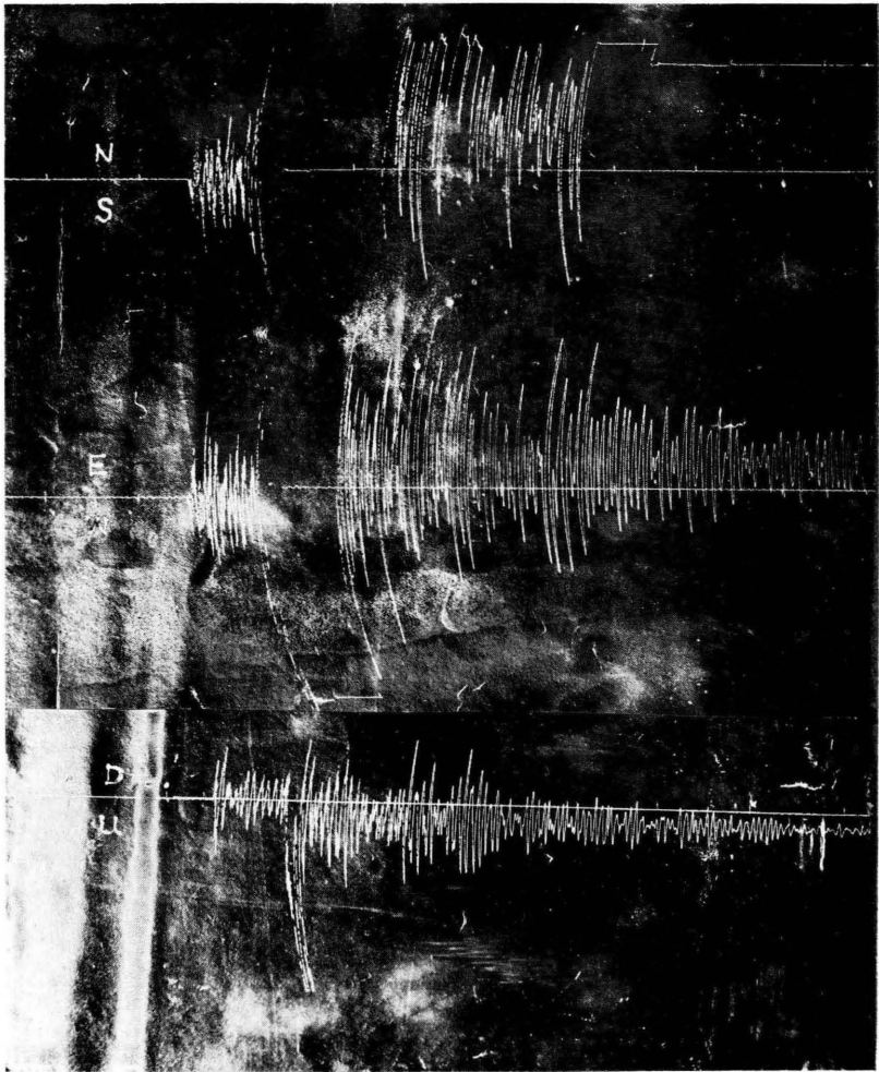
第一圖 志摩半島沖深發地震のワイーヘルト式地震計記象1 (短週期波の發達を示す) 中央氣象臺地震計室
