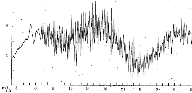
小名浜検潮儀記録
