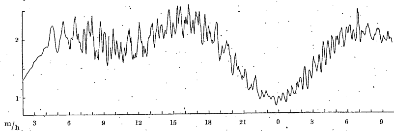
宮古檢潮儀記錄
