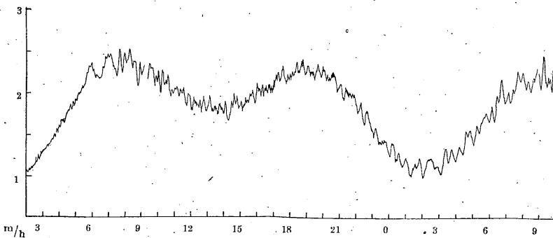
内浦検潮儀記録
