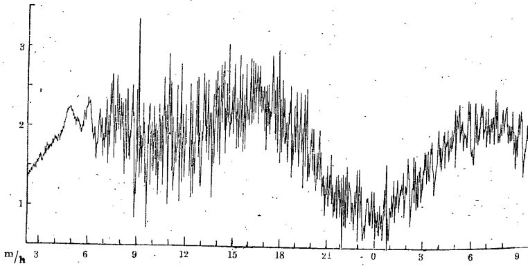
石巻検潮儀記録
