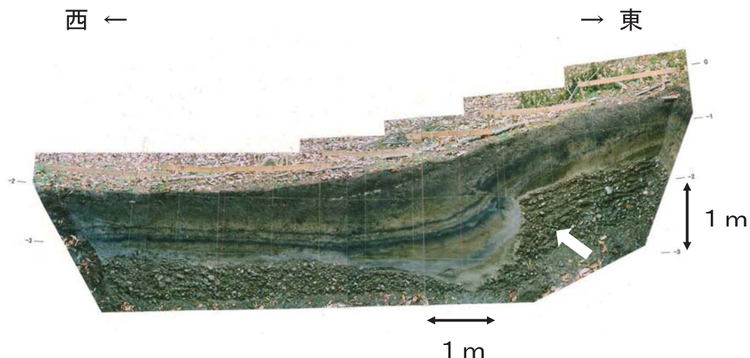
富良野断層帯（麗郷断層）のトレンチ調査（北海道富良野市） 穴を掘って見えている地層の断面の中、白矢印の箇所で、地層にずれが生じており、ここで断層面が直接確認できる。
