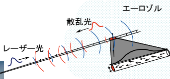
スキャナ部 散乱光の一部を スキャナで受ける
