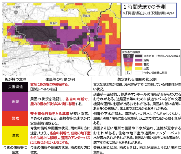
浸水キキクルの例
