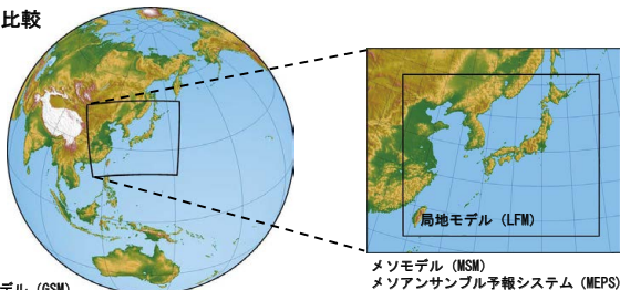
全球モデル (GSM) 全球アンサンブル予報システム (GEPS)
