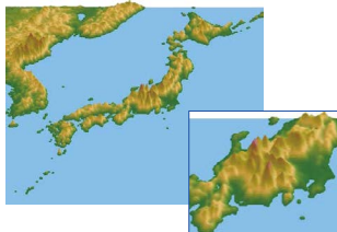
MSM, MEPS (格子間隔: 5km) の地形
